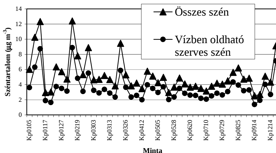
3.3 ábra Az összes szén és a vízoldható szerves szén koncentrációja a 2000-ben K-pusztán gyűjtött aeroszolmintákban.
