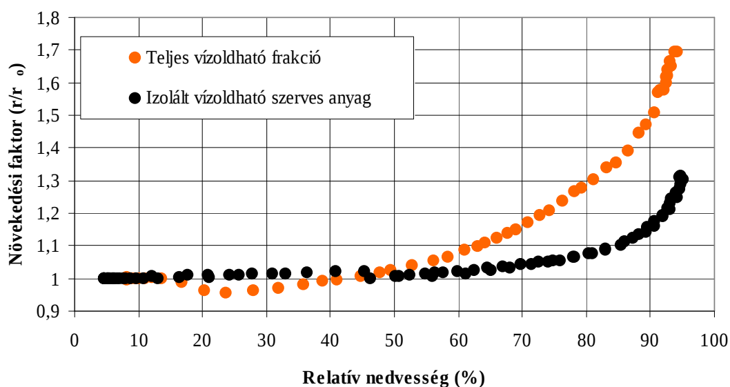
3.9 ábra A Kp010816 mintából izolált vízdoldható szerves anyag és az összes vízdoldható anyag higroszkópos növekedése
