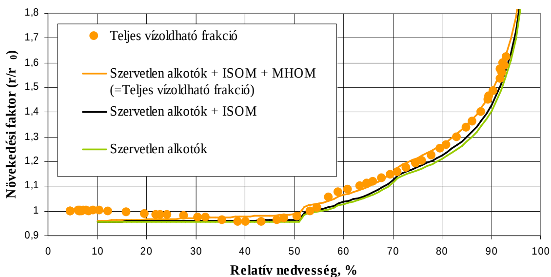
3.10 ábra A három vízoldható frakció (ISOM=izolált vízoldható szerves anyag, MHOM=nem izolált hidrophil szerves anyag) együttes hatásának modellezése és összehasonlítása a mérési eredményekkel a Kp010112 minta esetében
