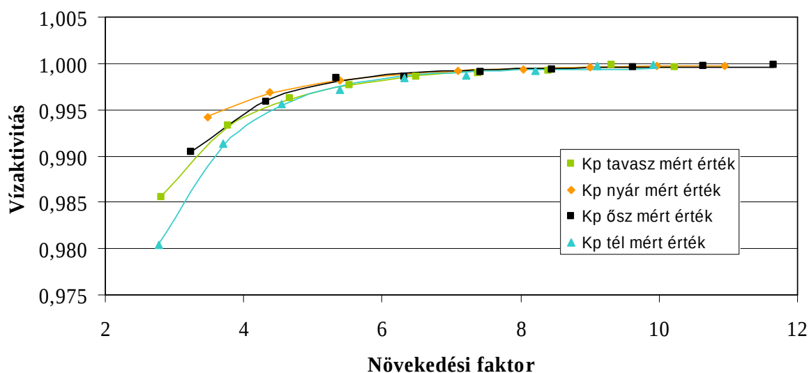
3.21 ábra A K-pusztán gyűjtött légköri aeroszol minták és a biomassza égetésből származó minták vízaktivitása a növekedési faktor függvényében
