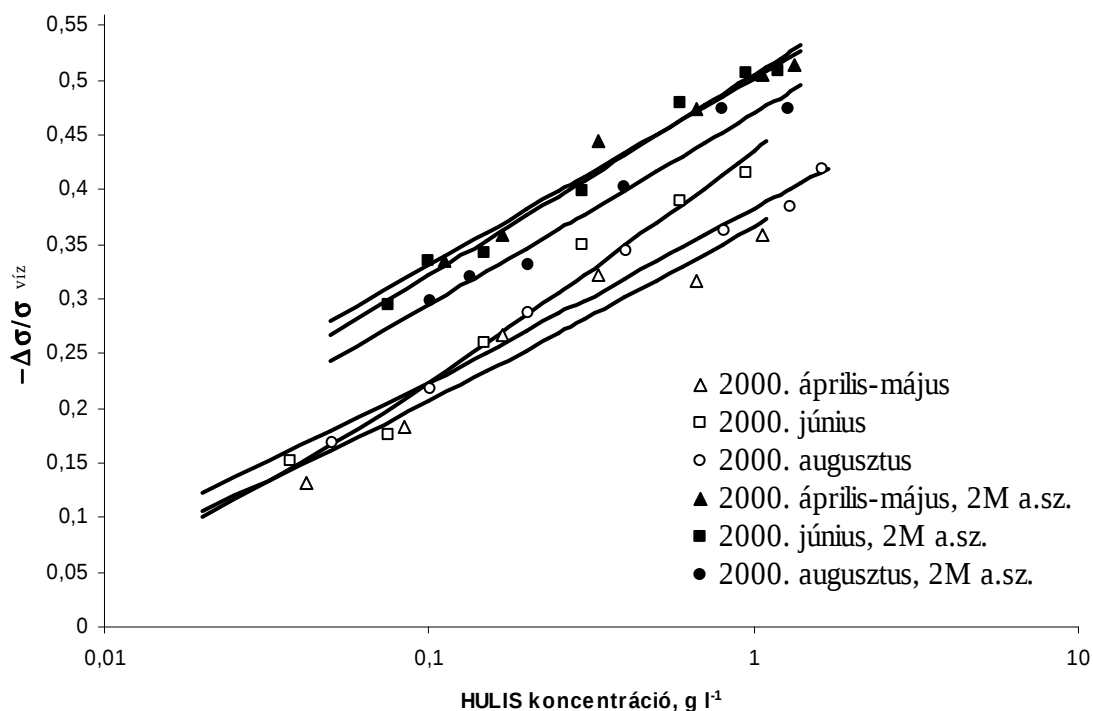
3.12 ábra A K-pusztán gyűjtött finom aeroszorból izolált vízzoldható szerves anyag felületi feszültség csökkentő hatása a koncentráció függvényében, 2M ammónium-szulfát oldatban, illetve anélkül. Az ábrán az „a.sz.” felirattal az ammónium-szulfátot rövidítettem.
