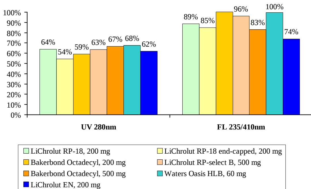
3.1 ábra: A.) A vízben oldható szerves szén kinyerése a hét vizsgált oszloppal; B.) A különböző oszlopokkal kinyert szerves anyag hozzájárulása az eredeti vizes extraktum UV elnyeléséhez (280 nm) és fluoreszcenciás aktivitásához (gerjesztés: 235nm, emisszió: 410 nm)
