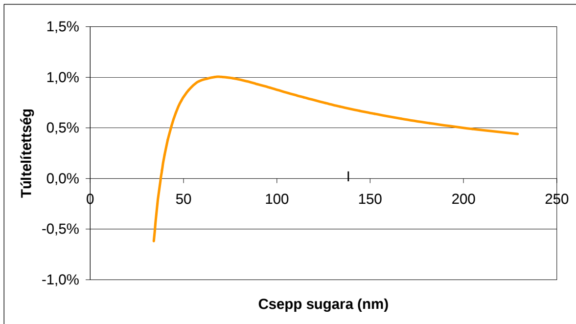
1.3 ábra A 15 nm sugarú ammónium-szulfát részecske Köhler görbéje
