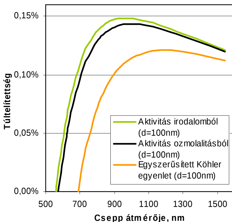
3.16 ábra Az eredeti Köhler egyenlettel (irodalmi, illetve ozmolalitásból származtatott aktivitással) és az egyszerűsített egyenlettel 100 nm-es kénsav cseppre számított Köhler görbék
