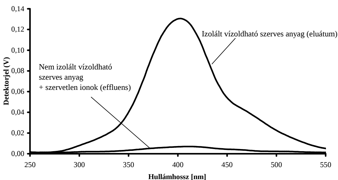
3.5 ábra Léggöri finom aeroszol vizes extraktumából folyadék-szilárd extrakcióval nyert két frakció fluoreszcens emissziós spektruma (gerjesztés: 235nm)
